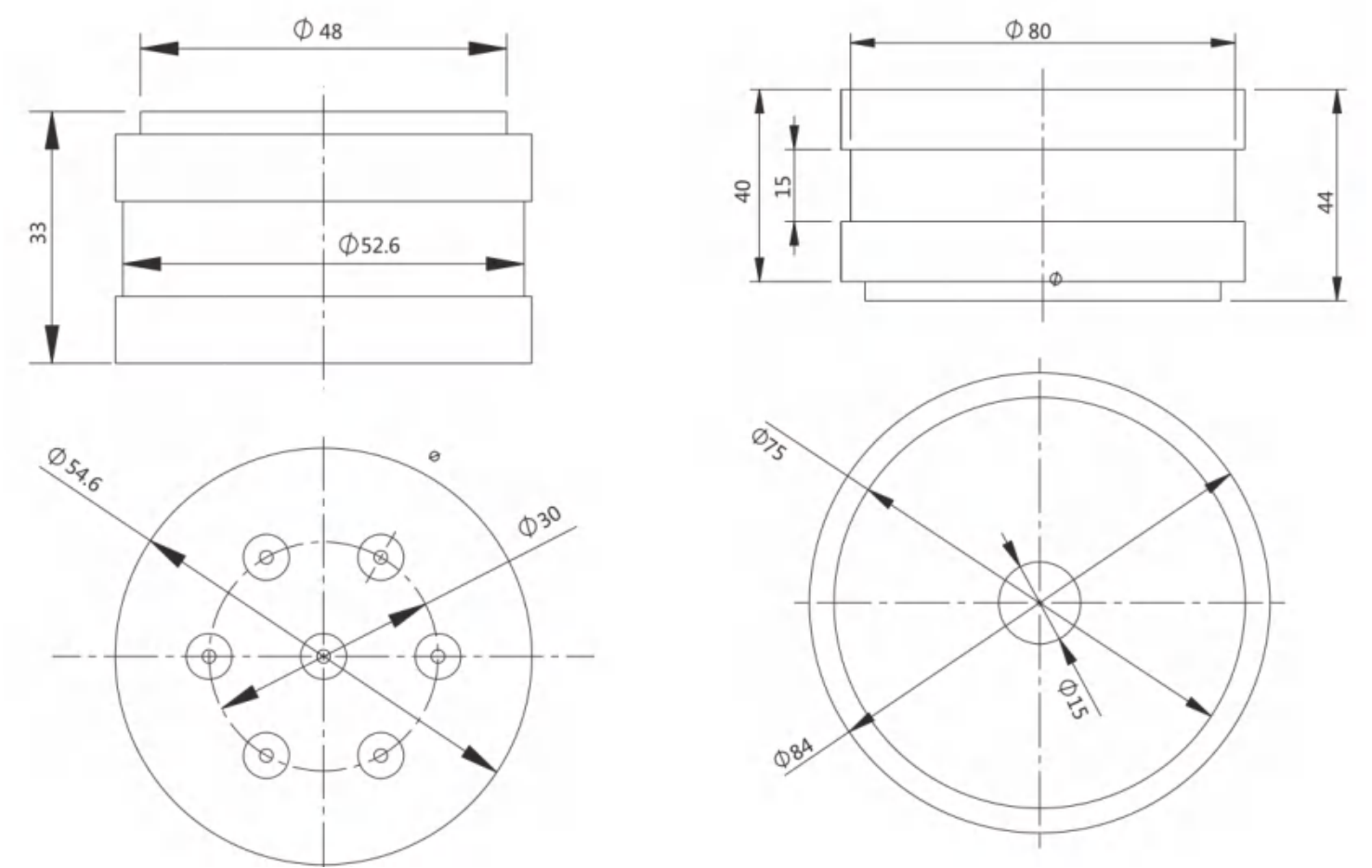
RGFX外形图
