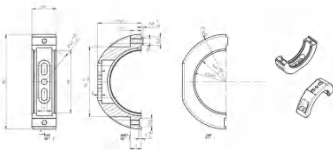
RGLV-70尺寸图2
