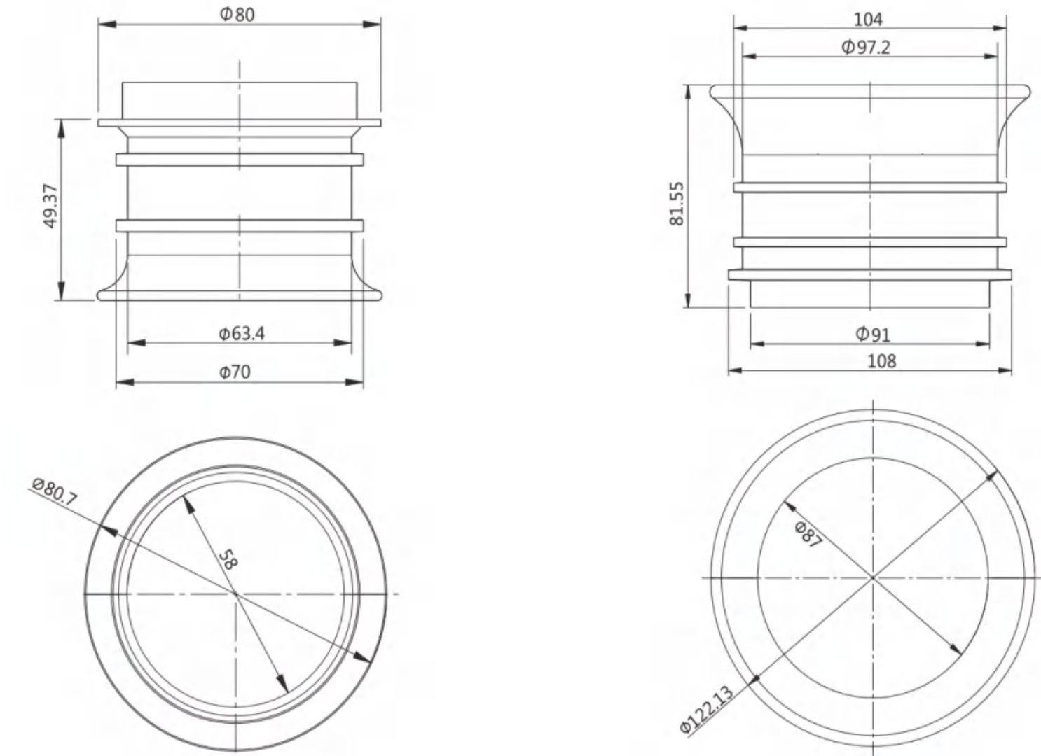
RGDX导向套筒外形图
