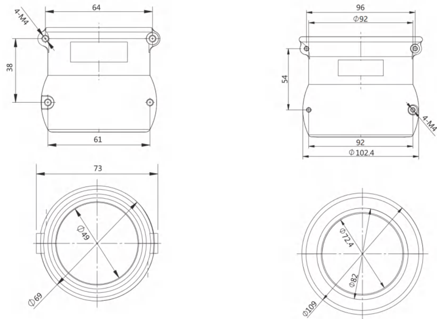
RGMD外形图
